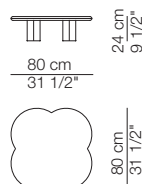
Tavolino 80 x 80 H.24 cm Small table 80 x 80 H.24 cm
